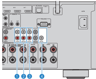
L'unité (arrière)
