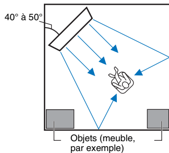
Installation en angle : Vue du dessus
