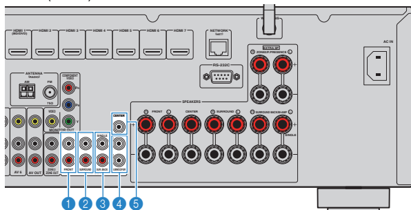
L'unité (arrière)
