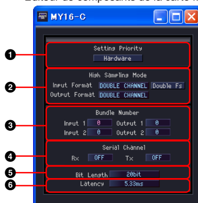
Editeur de composants de la carte MY16-C
