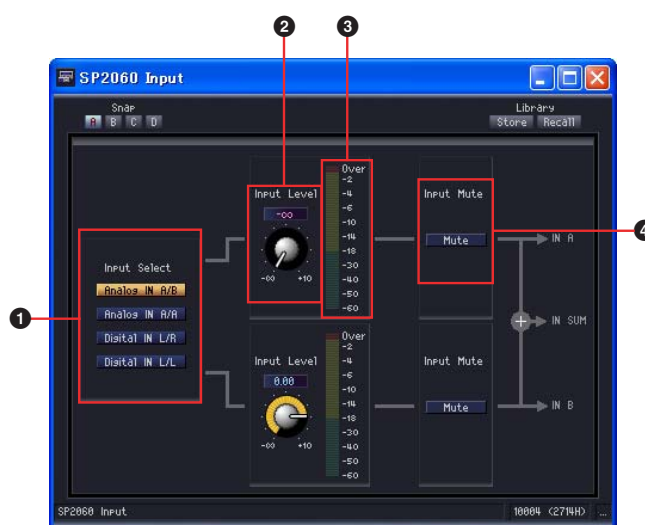
SP2060 Input Component Editor (Editeur de composants d'entrée SP2060)
