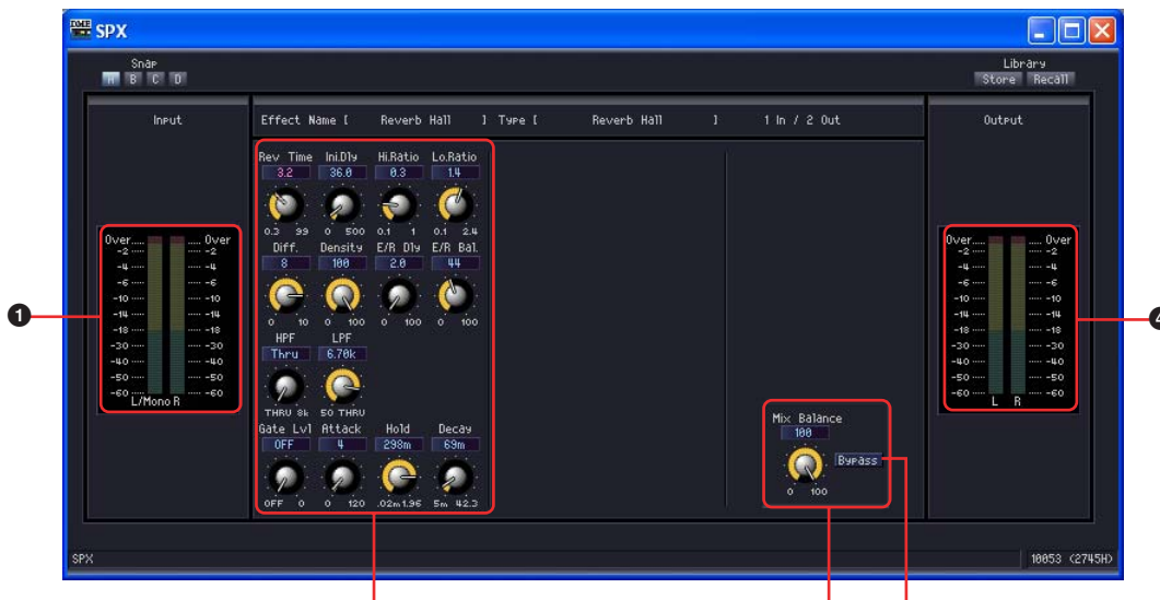
Editeur du composant SPX
