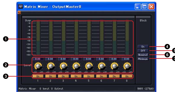
Fenêtre [Matrix Mixer - OutputMaster] de l'éditeur
