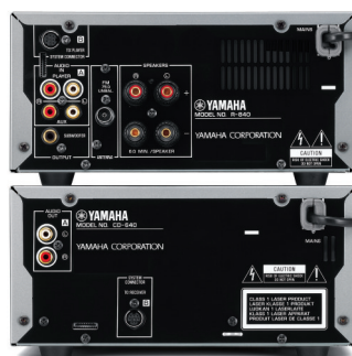
Vue arrière
